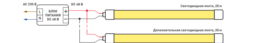
Схема 1. Подключение нескольких светодиодных лент «неон» с одной стороны
